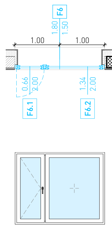
F6: FINESTRA 180*150
