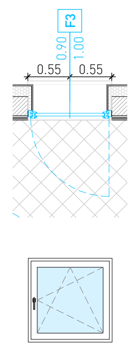
F3: FINESTRA 90*100
