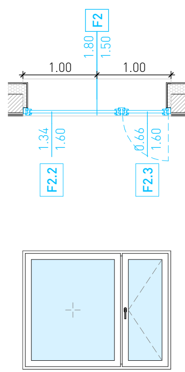
F2: FINESTRA 180*150
