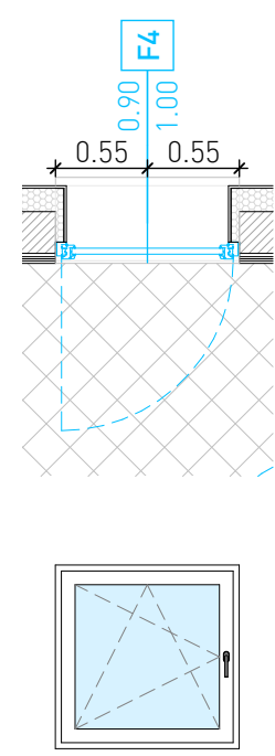
F4: FINESTRA 90*100
