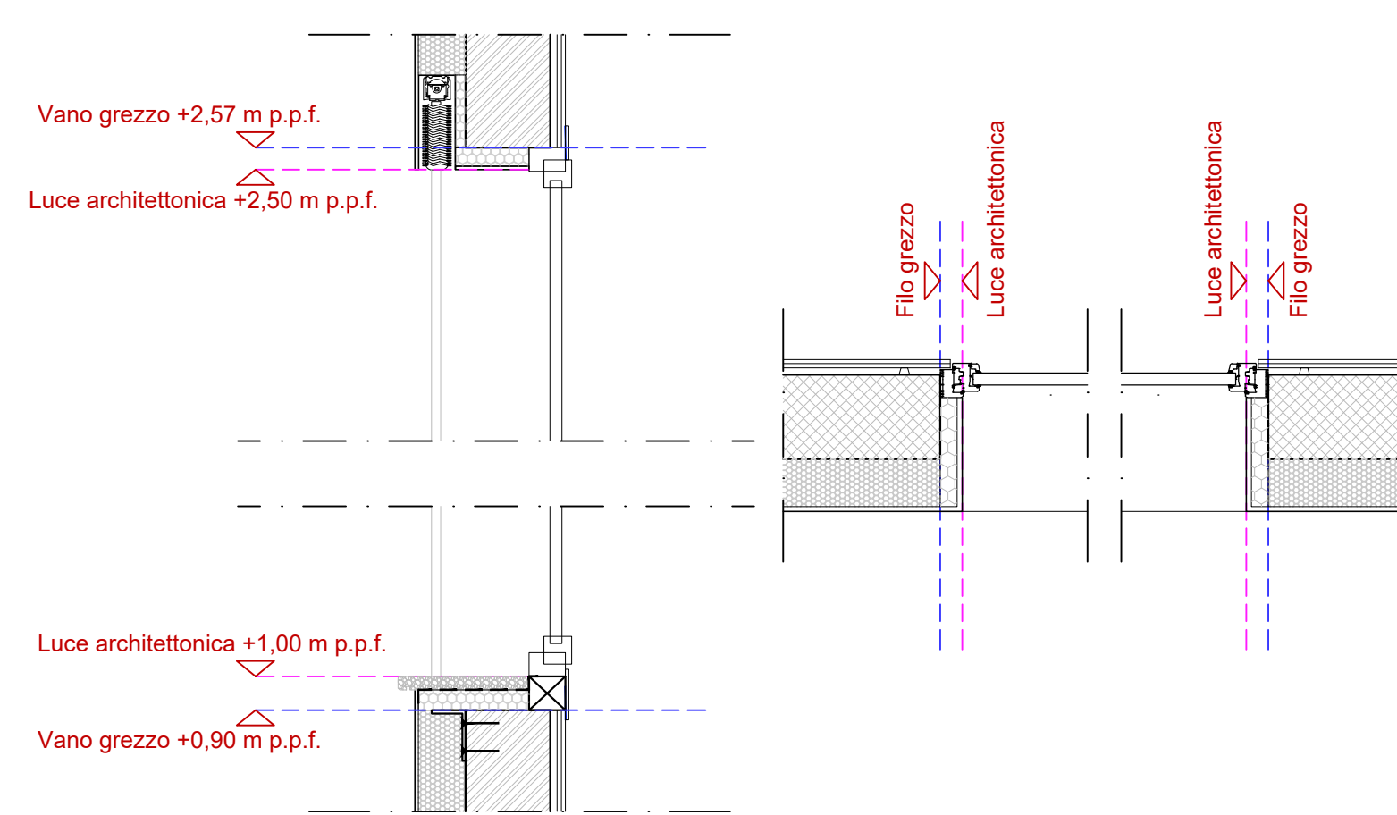
DETTAGLIO SERRAMENTO: scala 1:20
