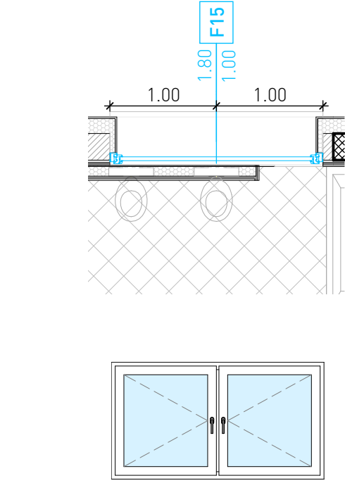
F15: FINESTRA 180*100
