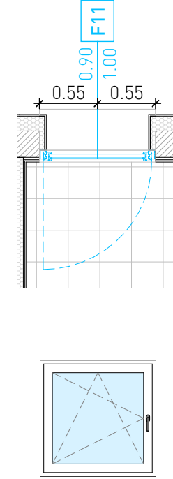
F11: FINESTRA 90*100
