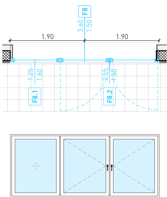
F8: FINESTRA 360*150
