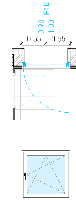
F10: FINESTRA 90*100
