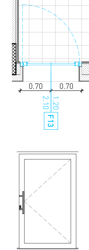
F13: PORTA LOCALE TECNICO 120*210
