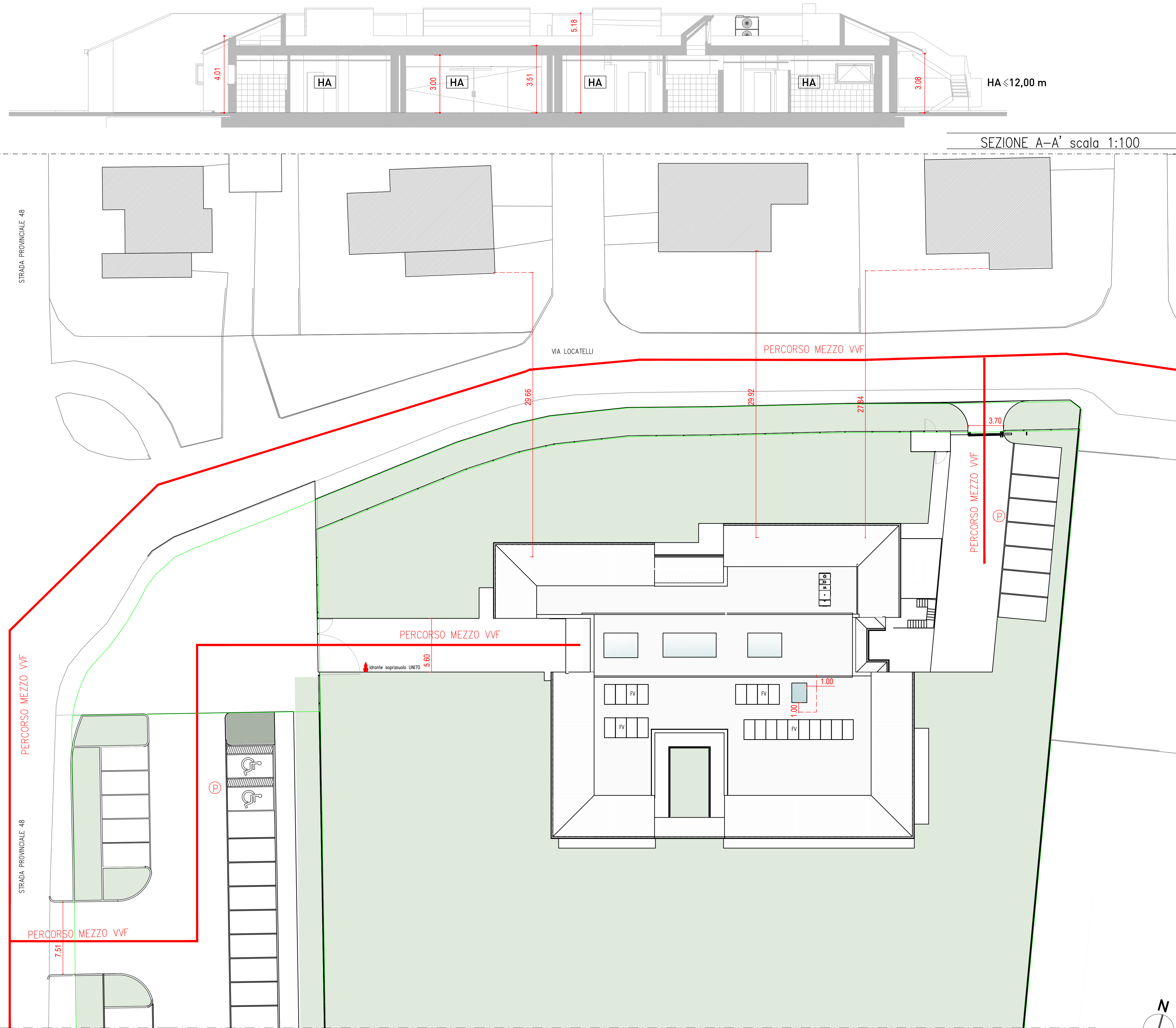
PIANTA GENERALE AVVICINAMENTO MEZZI V.F.
