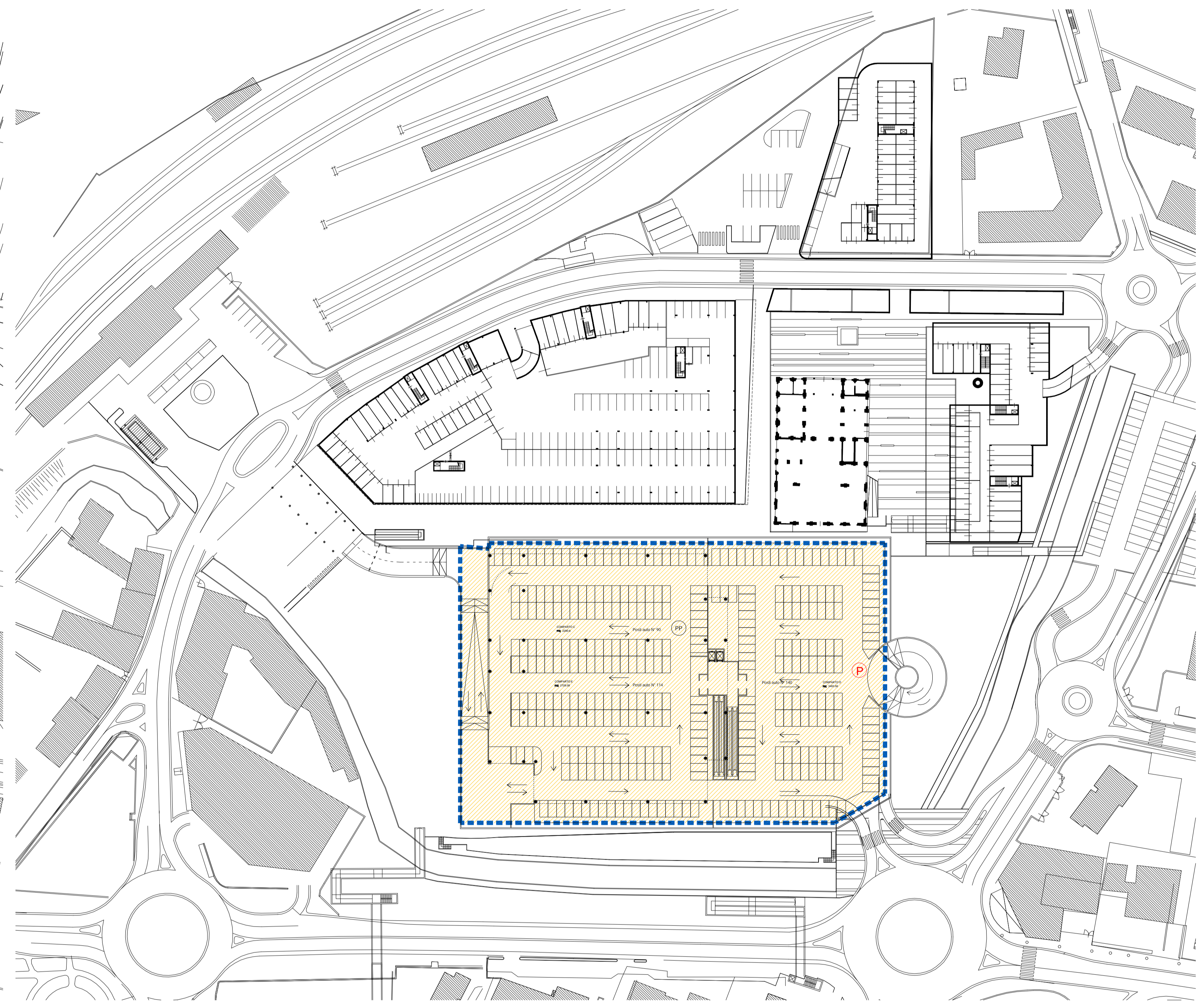
planimetria dei piani interrati
